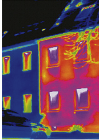
Ein Thermogramm von zwei Häusern zeigt, welches besser gedämmt ist.
